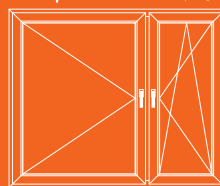
Dvojkrídlové plastové okno 1800 x 1500mm:
